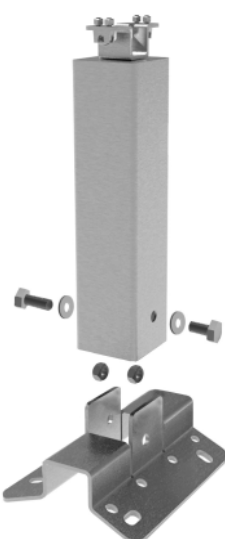
ANCORAGGIO TIPO C H45/60 cm PIASTRA COLMO CON BLOCCO FUNE
