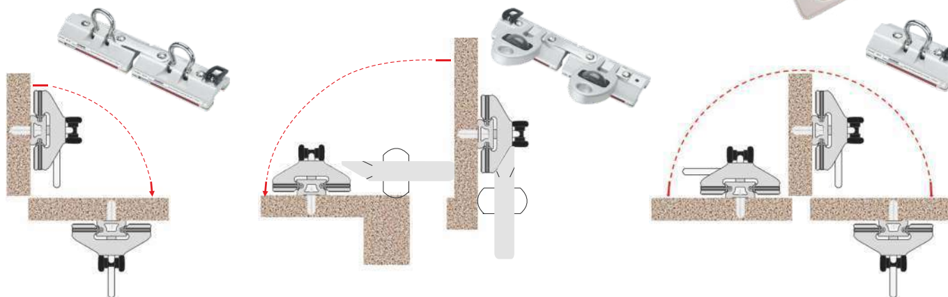
Posizionamento binario e relativo carrello
